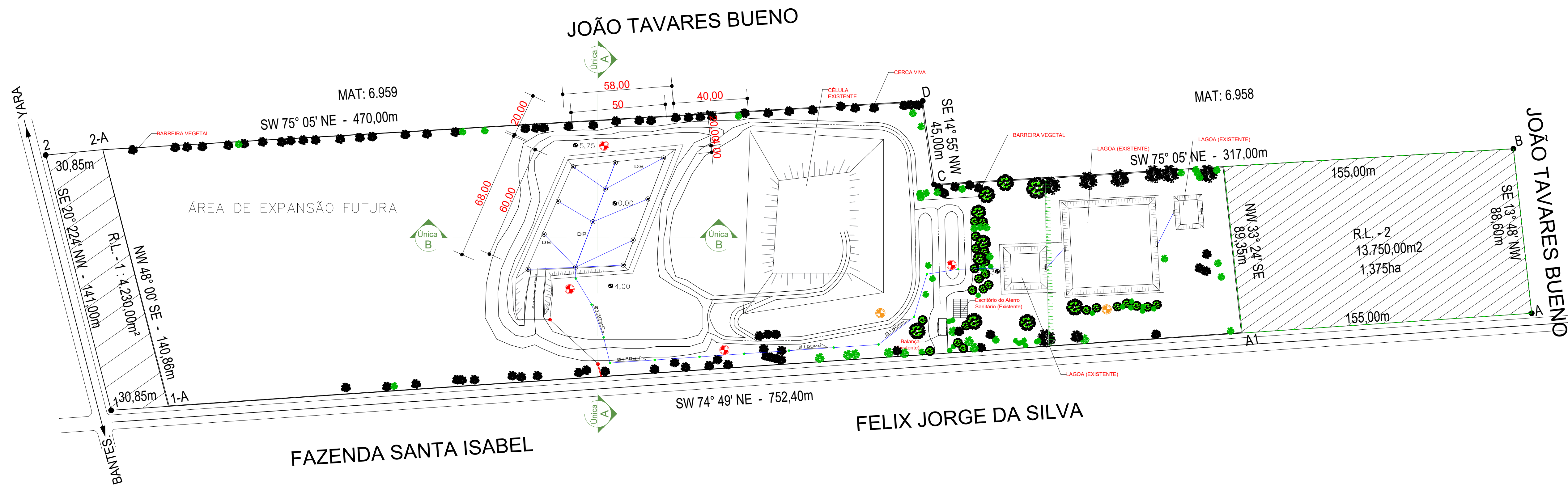
4 LEVANTAMENTO TOPOGRÁFICO ESCALA - 1:1250
