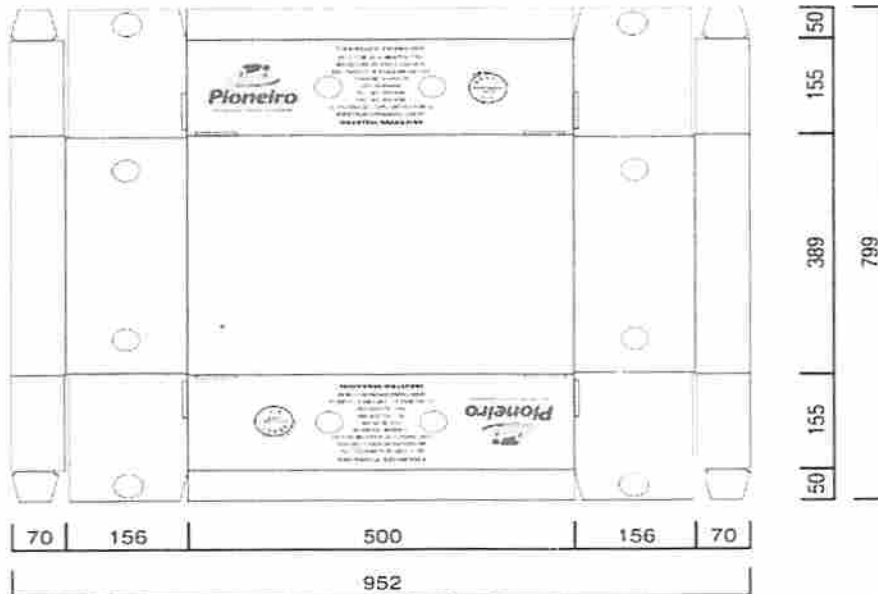
Medidas Externas (Caixa Montada)
