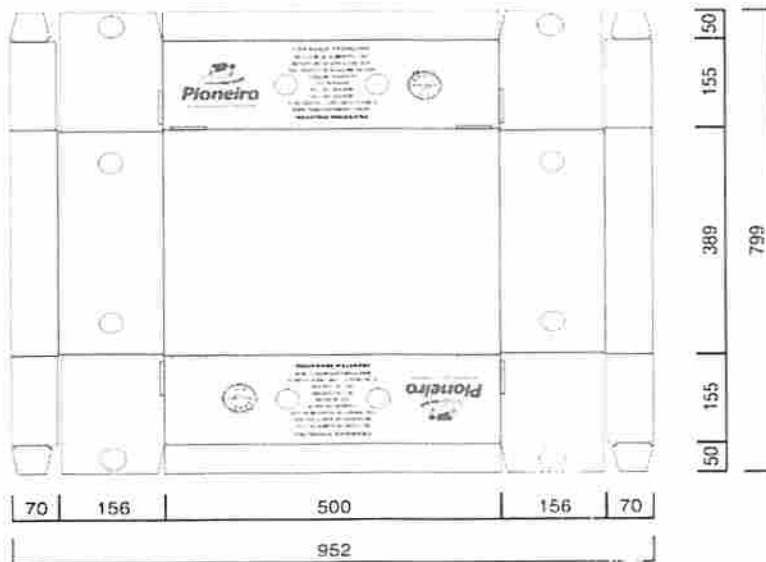
Medidas Externas (Caixa Montada)
