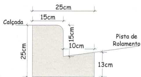
Detalhe meio fio e sarjeta Sem Escala
