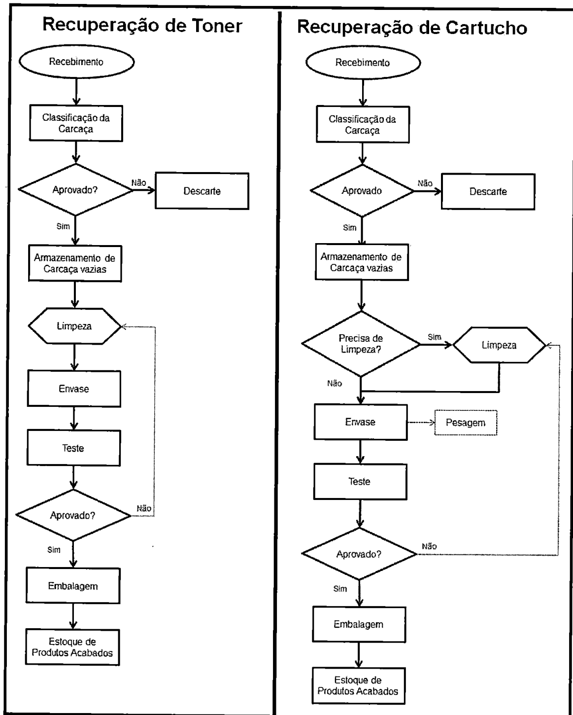
Figura 2 – Processo de reciclagem de Toners e Cartuchos.
